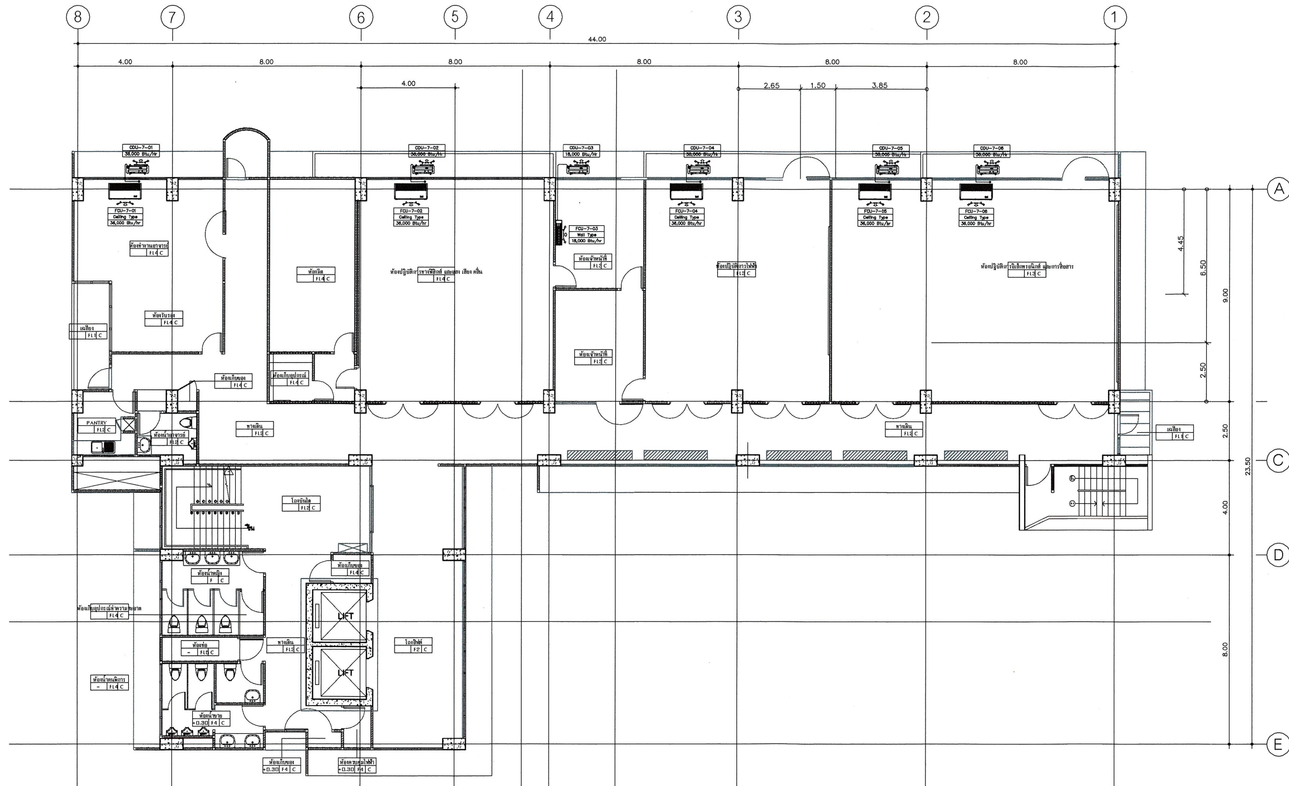
แปลนพื้นที่ชั้นที่ 7 (แบบตำแหน่งติดตั้งเครื่องปรับอากาศชั้นที่ 7) มาตราส่วน 1:75
