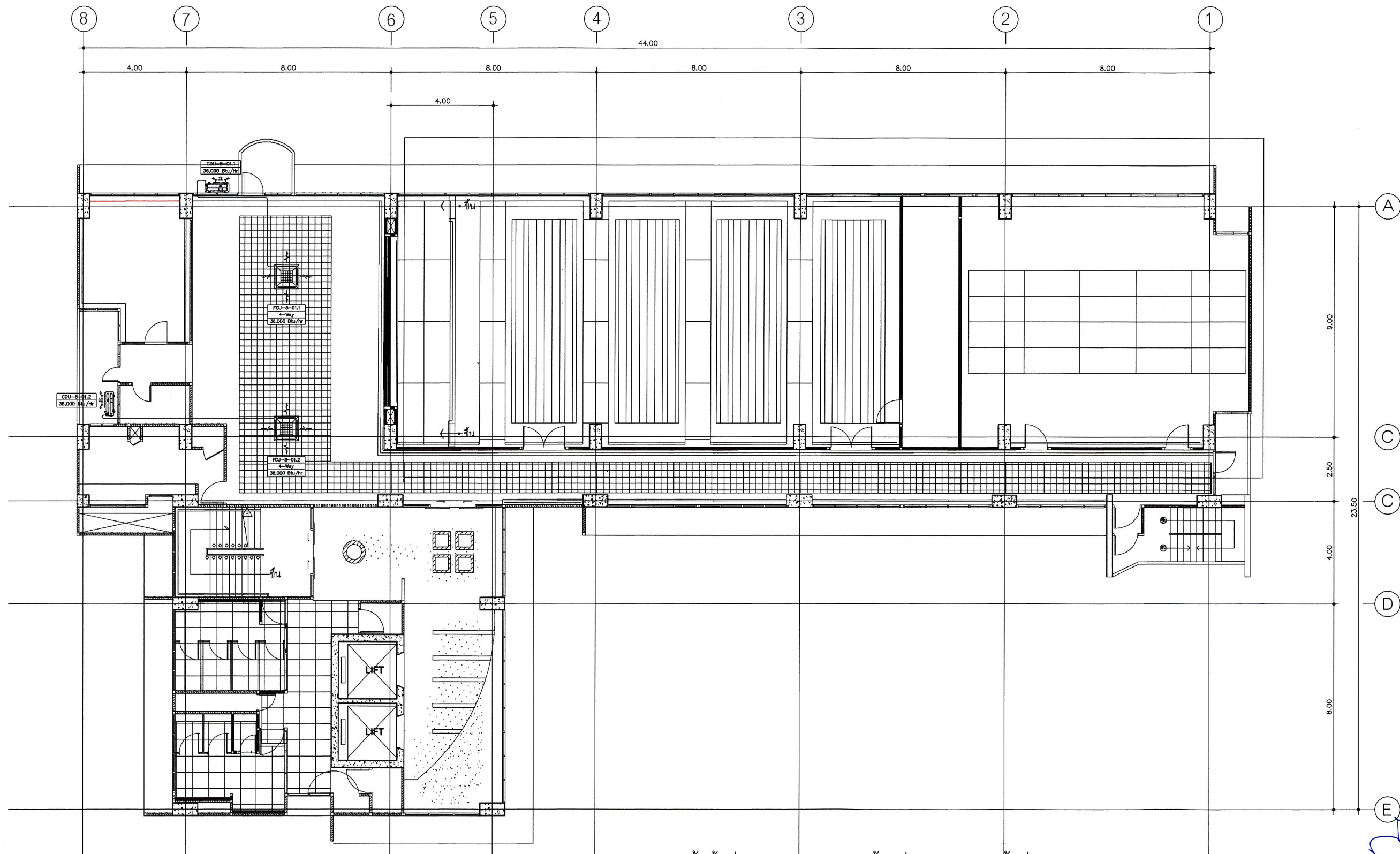
แปลนพื้นที่ 8 (แบบตำแหน่งติดตั้งเครื่องปรับอากาศพื้นที่ 8) มาตราส่วน 1:75
