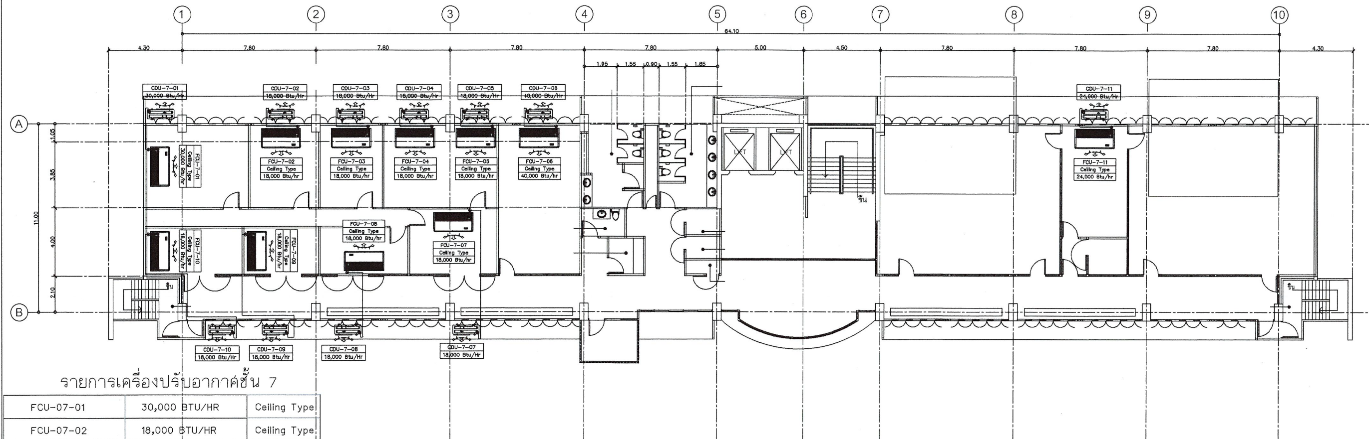
แปลนพื้นที่ 7 (ตำแหน่งติดตั้งเครื่องปรับอากาศชั้น 7)
