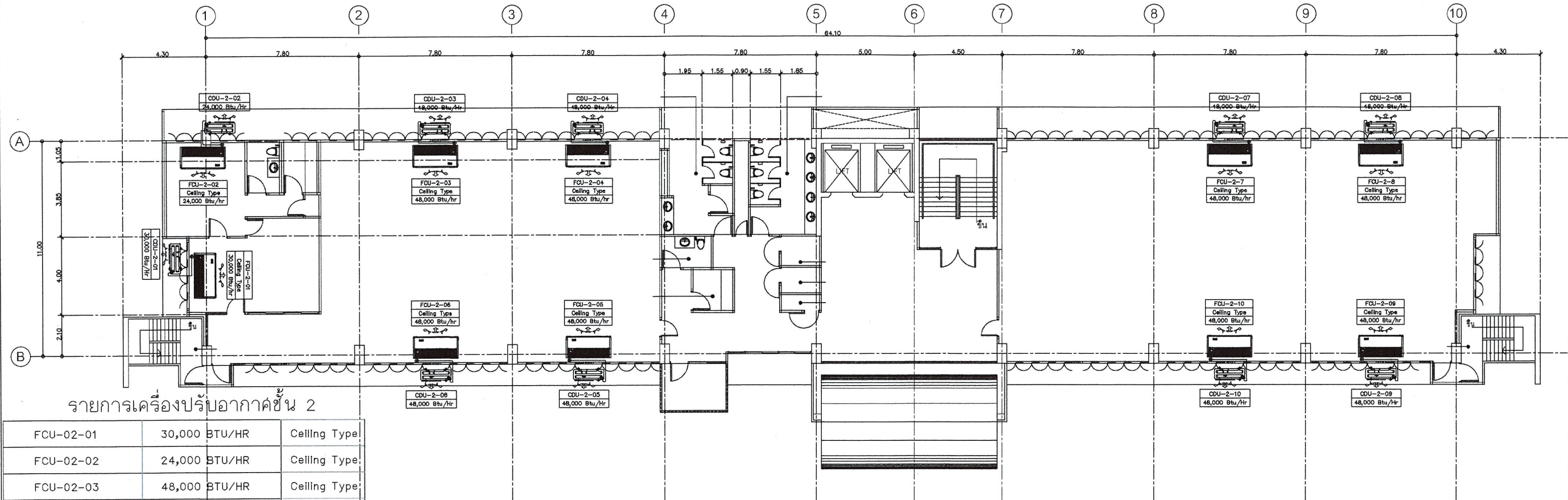
แปลนพื้นที่ 2 (ตำแหน่งติดตั้งเครื่องปรับอากาศชั้น 2) มาตราส่วน 1:150
