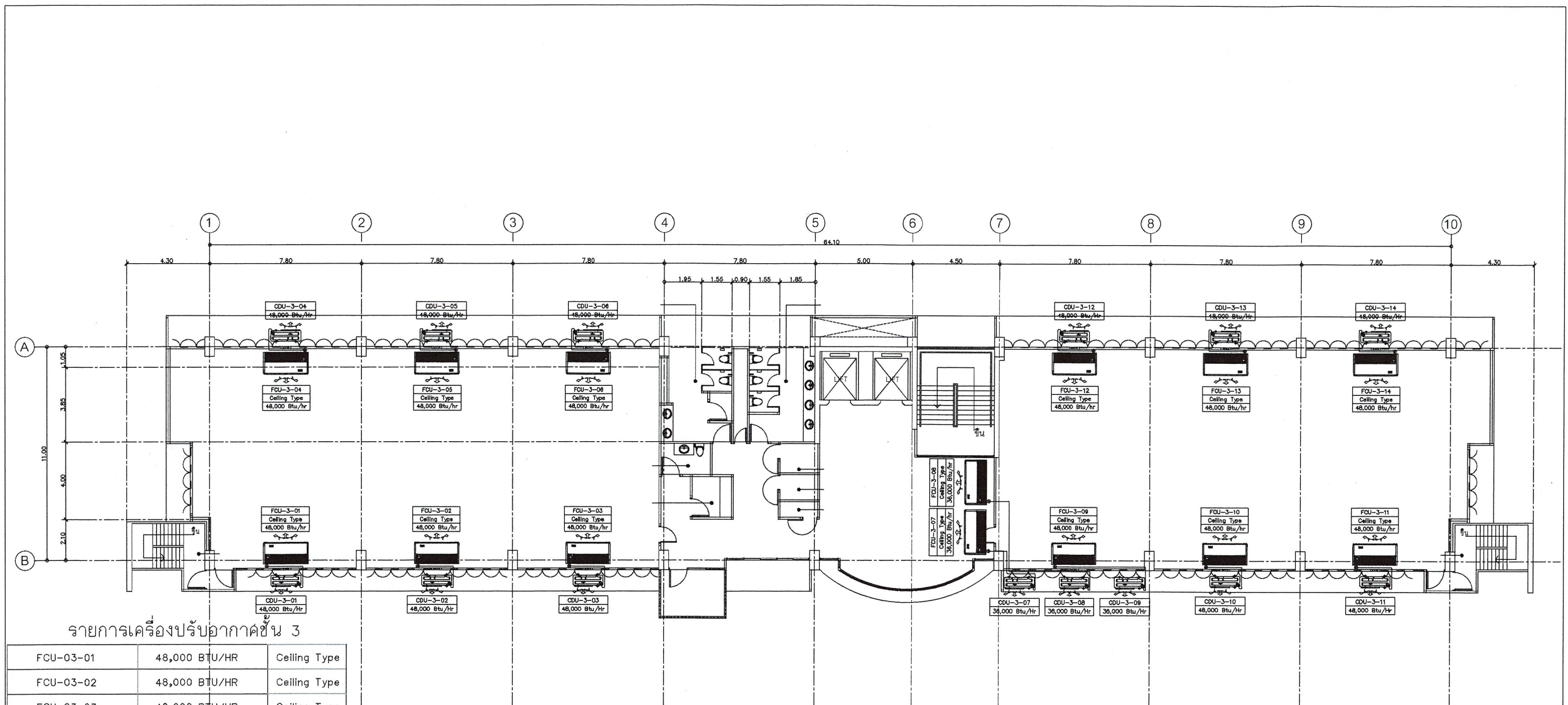
แปลนพื้นที่ 3 (ตำแหน่งติดตั้งเครื่องปรับอากาศชั้น 3)
