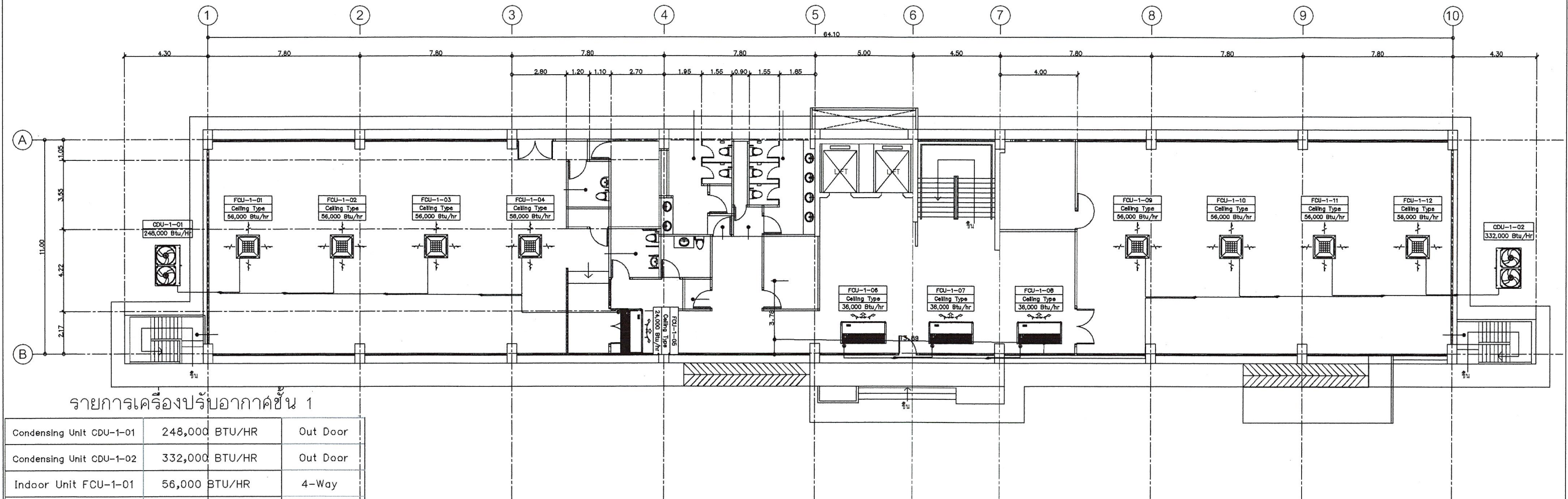
แปลนพื้นที่ 1 (ตำแหน่งติดตั้งเครื่องปรับอากาศชั้น 1) มาตราส่วน 1:150
