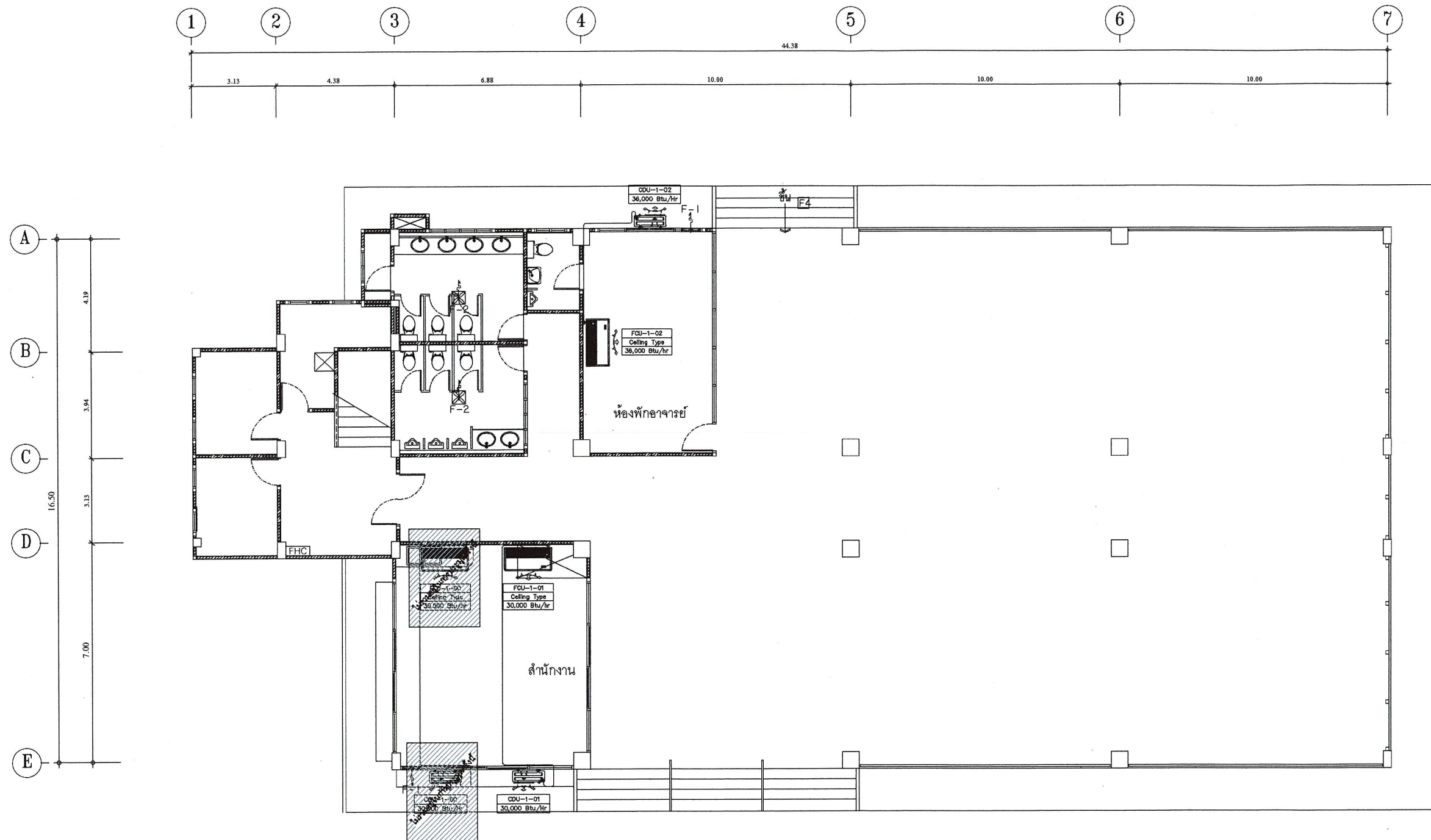
แปลนระบบปรับอากาศและระบายอากาศ ชั้นที่ 1 (1:100)
