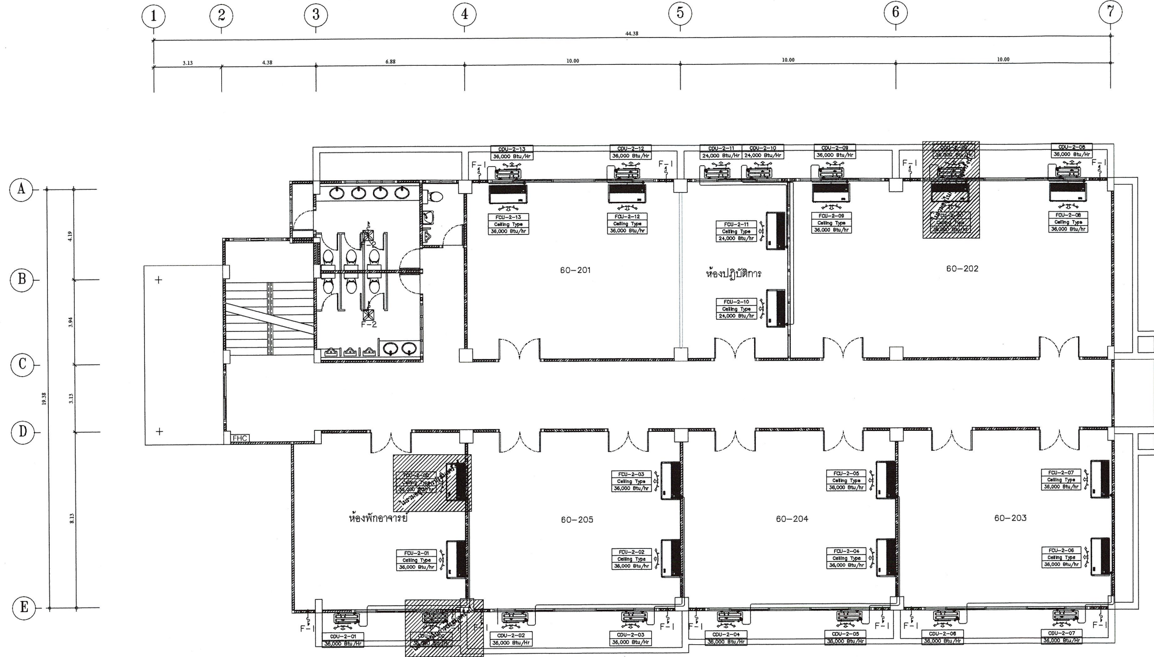
แปลนระบบปรับอากาศและระบายอากาศ ชั้นที่ 2 (1:100)
