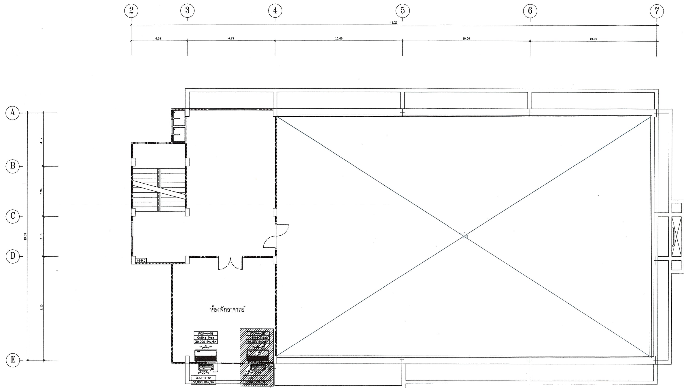
แปลนระบบปรับอากาศและระบายอากาศ ชั้นที่ 4 (1:100)
