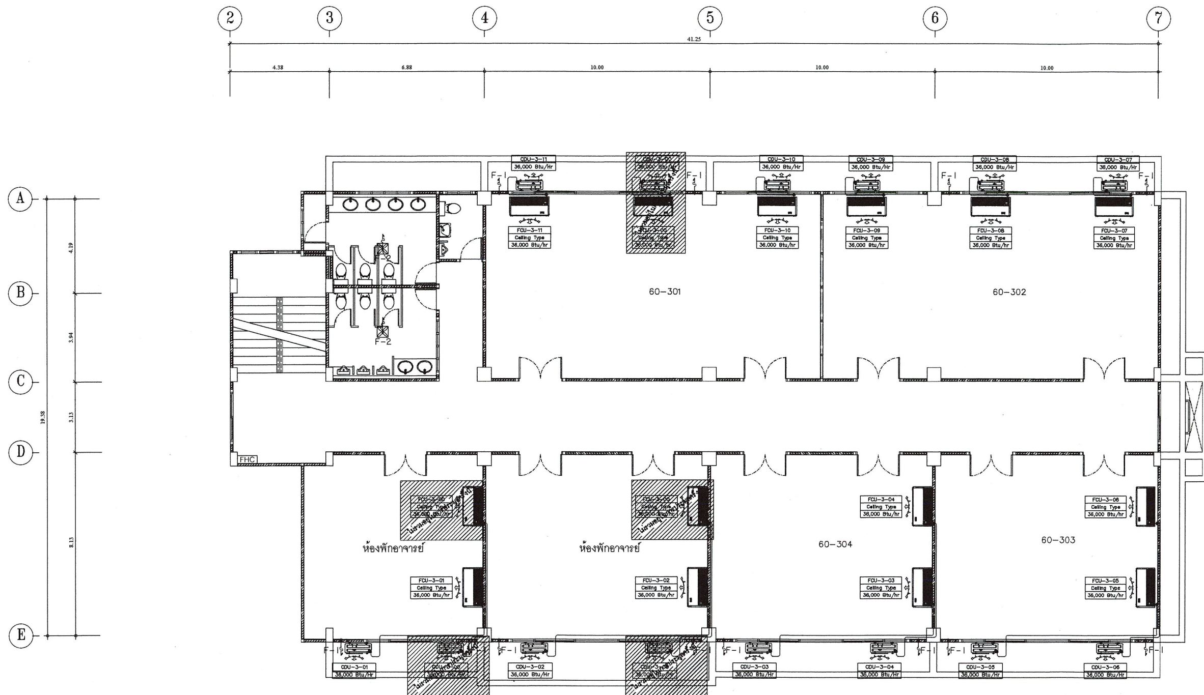
แปลนระบบปรับอากาศและระบายอากาศ ชั้นที่ 3 (1:100)
