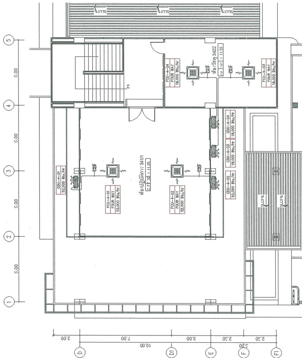
แบบแสดงตำแหน่งติดตั้งเครื่องปรับอากาศ ชั้นที่ 3 (ห้องปฏิบัติการ 341/1 และห้องสมุด 342/2)
