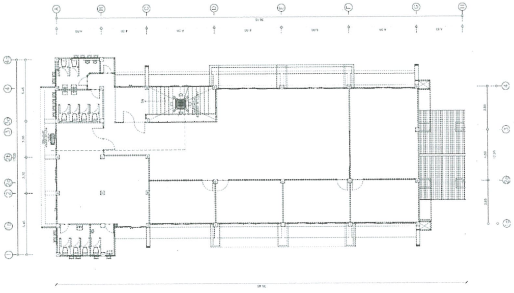
แปลนตำแหน่งเครื่องปรับอากาศ ชั้นที่ 2 1:1,100
