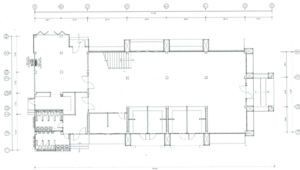
แปลนตำแหน่งเครื่องปรับอากาศ ชั้นที่ 1 1:1,100
