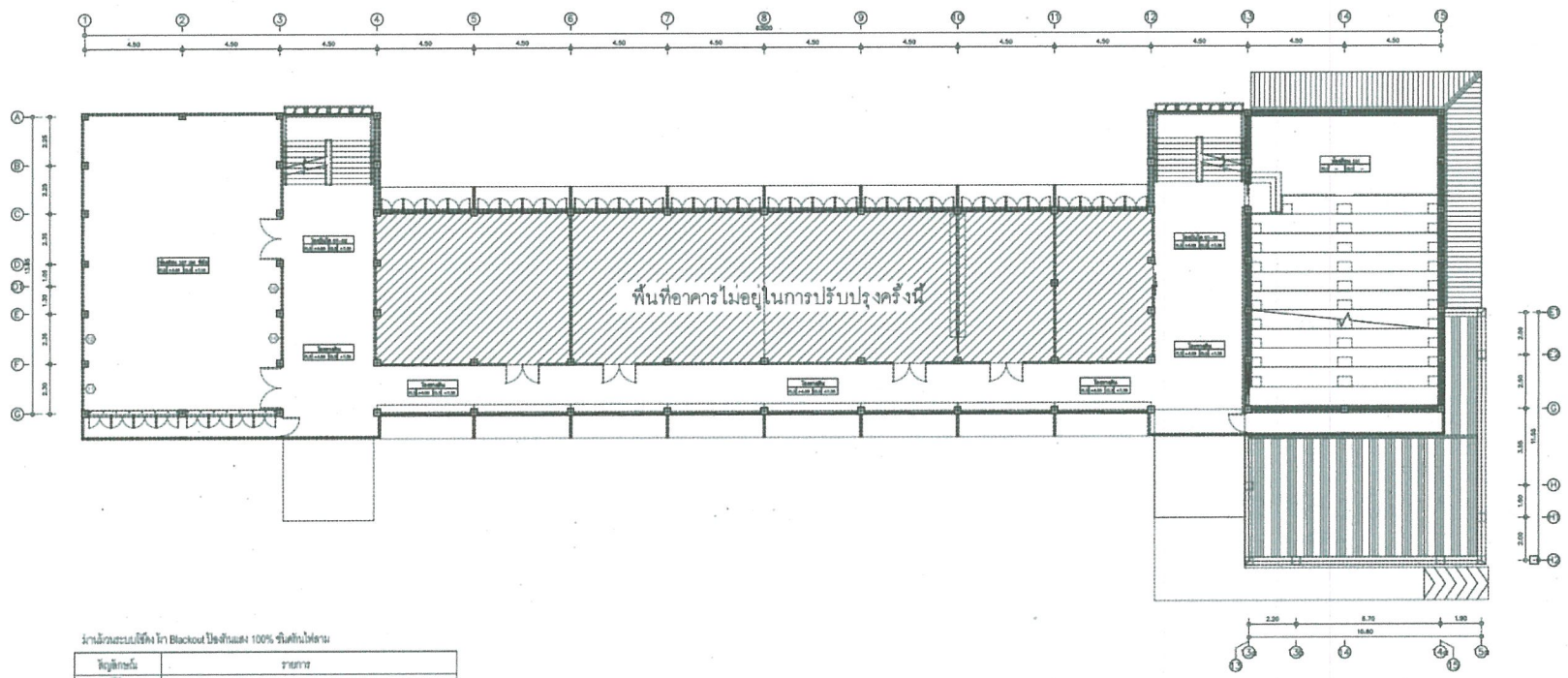
แปลนตำแหน่งครุภัณฑ์ผ้าม่านระบบโซติ่งชั้นที่ 2 มาตราส่วน 1:100
