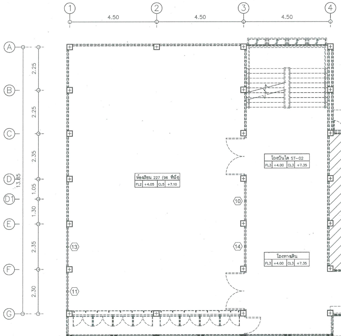
แปลนตำแหน่งครุภัณฑ์मानम्वनระบบโซ่ดิ่งชั้นที่ 2 (ห้องเรียน 227)
